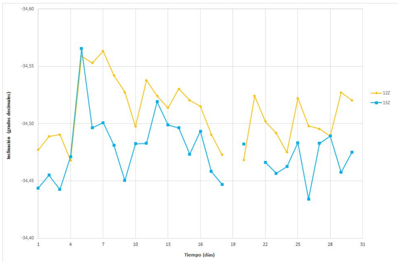
Figura 6: Inclinación magnética en función del tiempo
