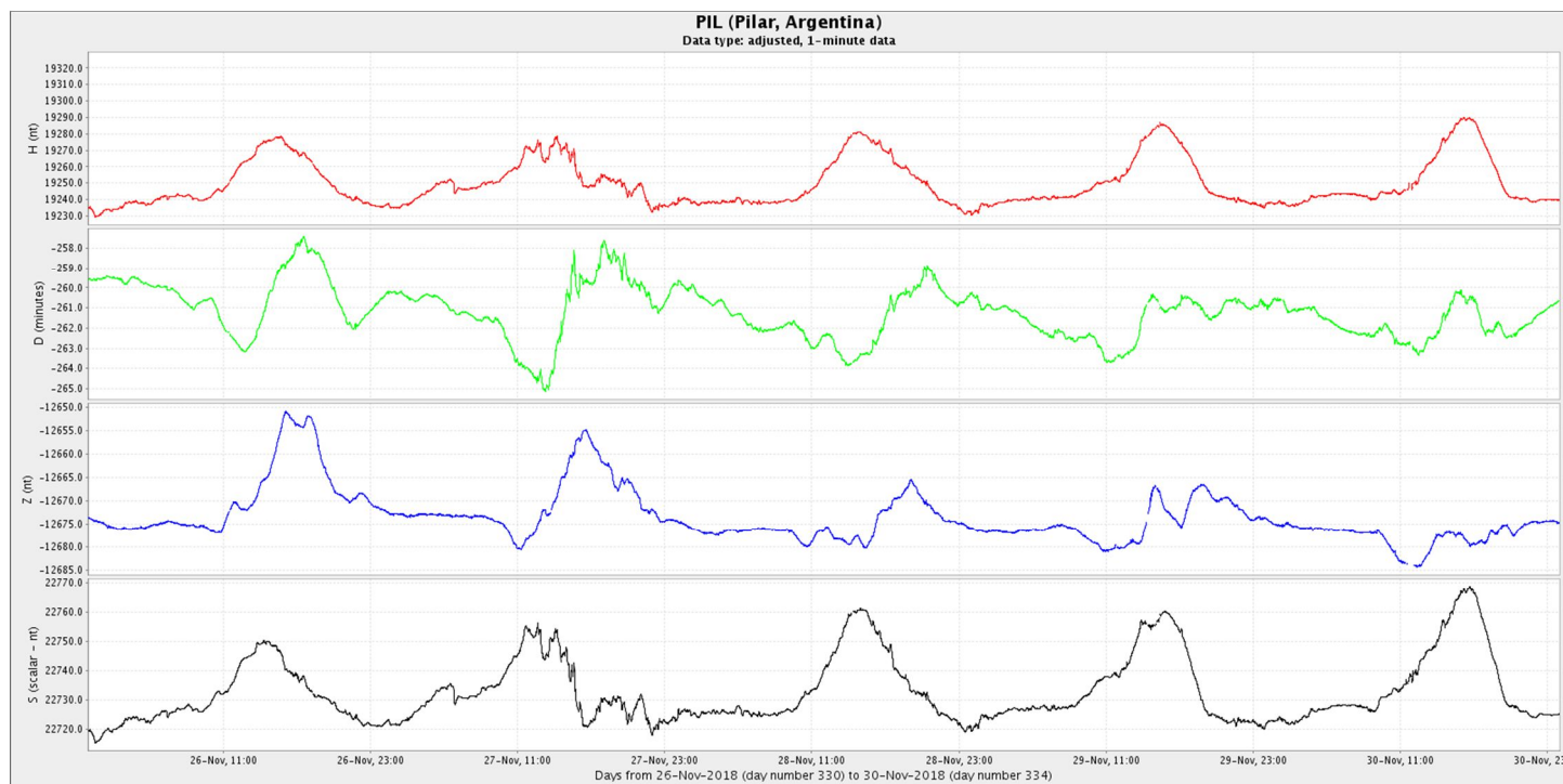
Figura 4c: Componentes del campo magnético del 21 al 30 de noviembre. En rojo se ve la componente horizontal ( H ) y en azul la vertical ( Z ), ambas en nT. En verde se presenta la declinación del campo magnético ( D ) en minutos y en negro la intensidad del campo magnético en nT.
