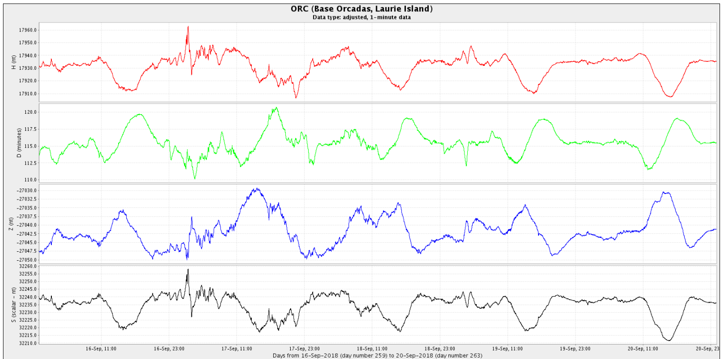
Figura 4b: Componentes del campo magnético del 11 al 20 de septiembre. En rojo se ve la componente horizontal ( H ) y en azul la vertical ( Z ), ambas en nT. En verde se presenta la declinación del campo magnético ( D ) en minutos y en negro la intensidad del campo magnético en nT.
