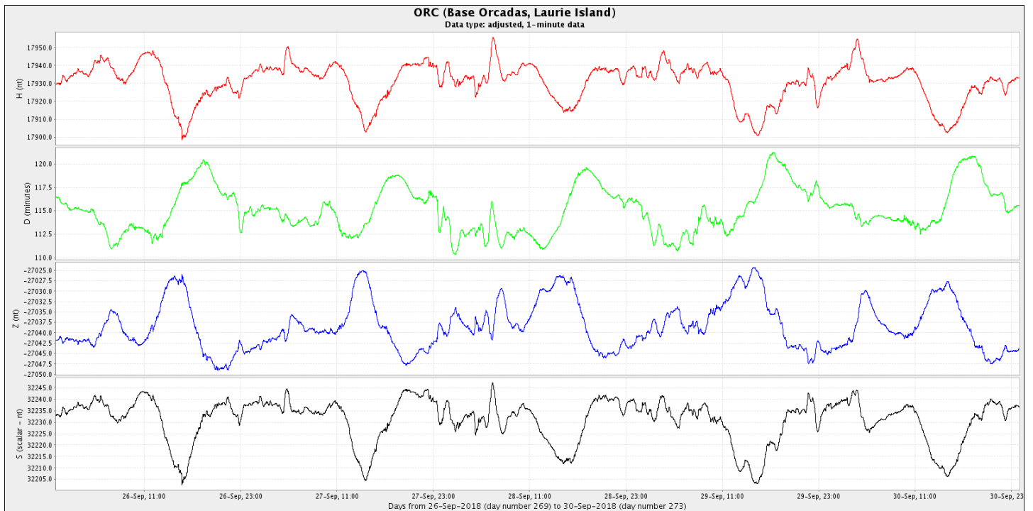
Figura 4c: Componentes del campo magnético del 21 al 30 de septiembre. En rojo se ve la componente horizontal ( H ) y en azul la vertical ( Z ), ambas en nT. En verde se presenta la declinación del campo magnético ( D ) en minutos y en negro la intensidad del campo magnético en nT.
