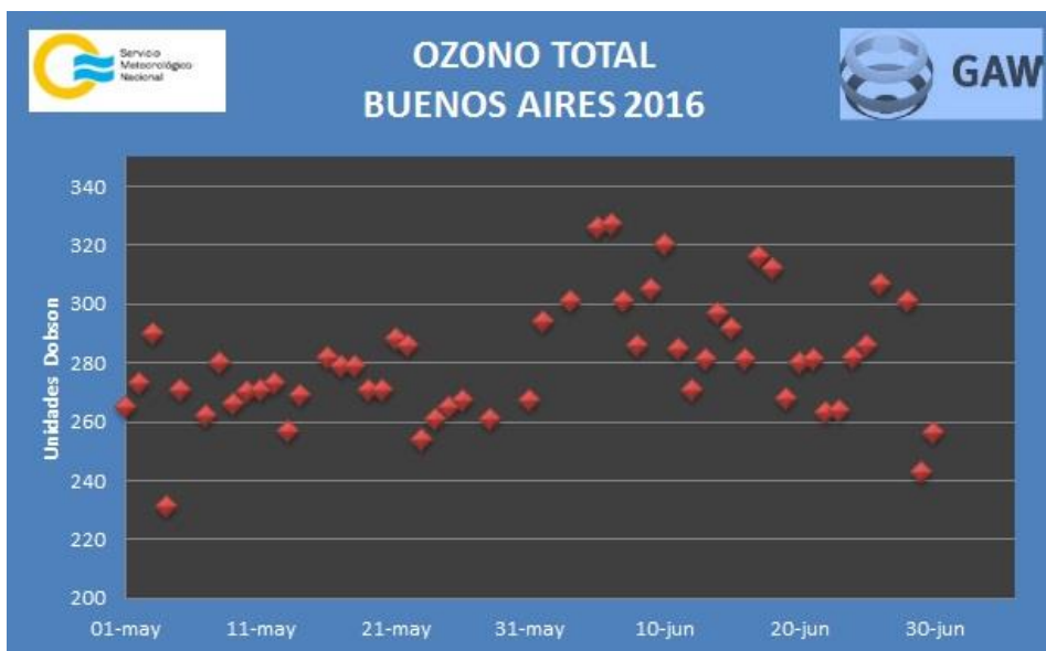
Figura 15. Columna total de ozono medida en Buenos Aires.
