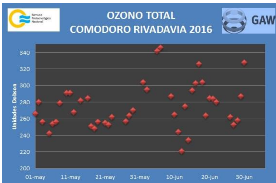
Figura 17. Columna total de ozono medida en Comodoro Rivadavia.
