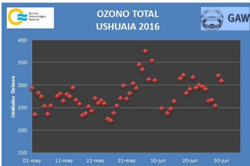
Figura 16. Columna total de ozono medida en Ushuaia.
