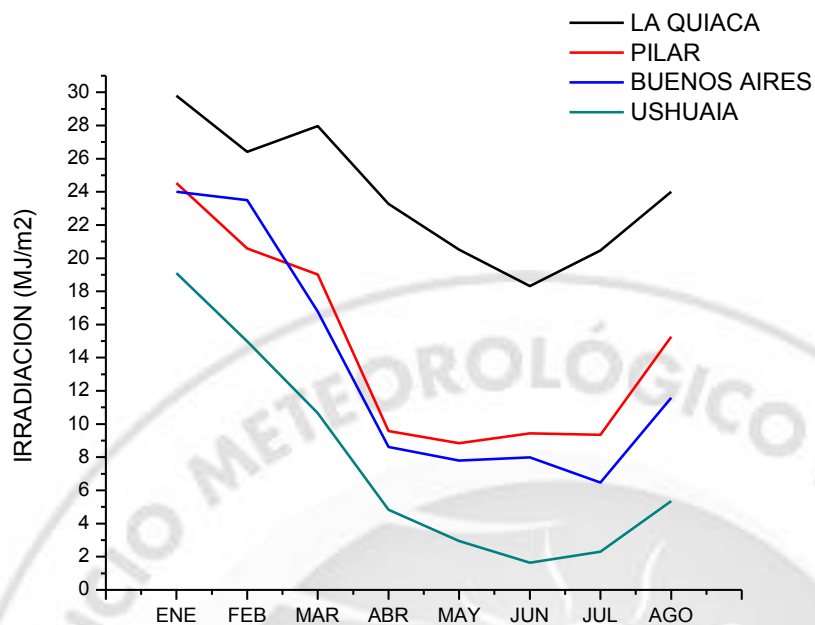
Figura 13. Promedio mensual de irradiación para cada lugar durante 2016.
