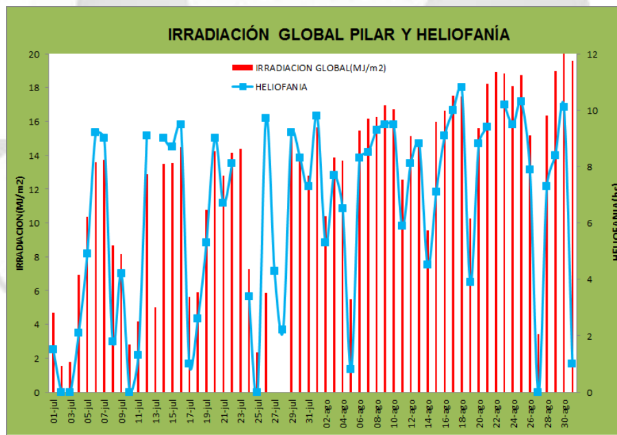
Figura 10. Heliofanía efectiva diaria junto con irradiación solar global diaria, ambas correspondientes a Pilar.
