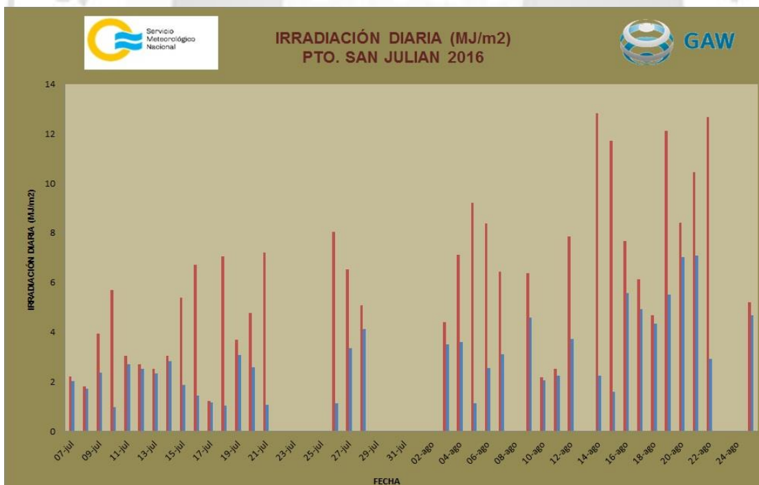
Figura 7. Irradiación global y difusa medida en Pto. San Julian.
