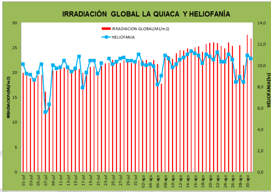
Figura 9. Heliofanía efectiva diaria junto con irradiación solar global diaria, ambas correspondientes a La Quiaca.
