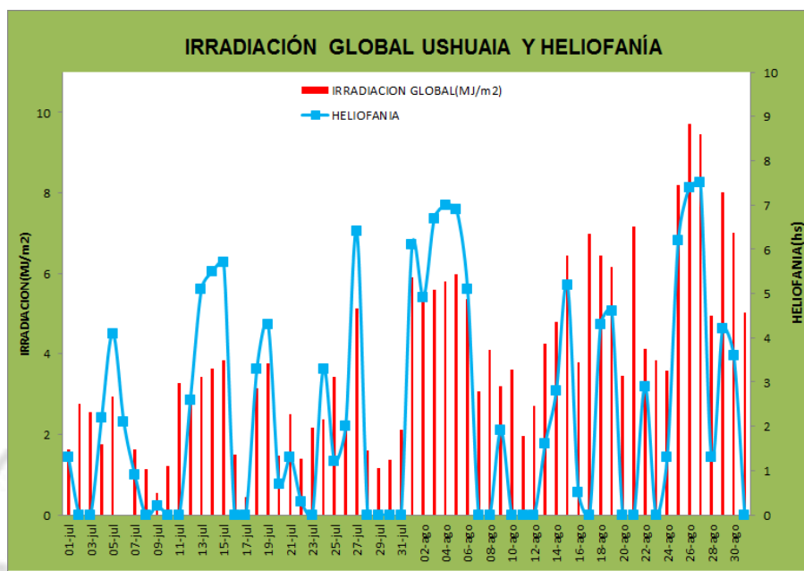
Figura 11. Heliofanía efectiva diaria junto con irradiación solar global diaria, ambas correspondientes a Ushuaia.
