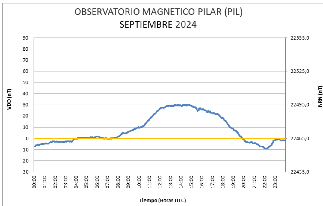
Figura 8: Variación Diaria Calma del mes de septiembre
