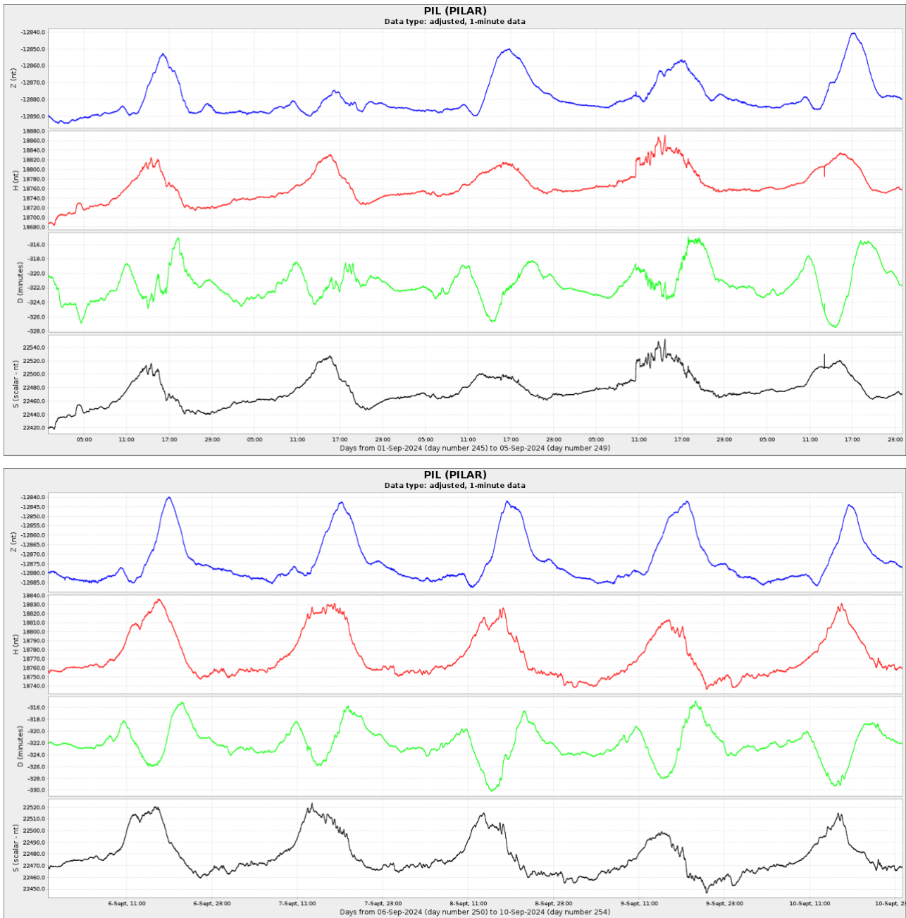
Figura 4a: Componentes del campo magnético del día 1 al 10 de Septiembre. En rojo se ve la componente horizontal (H) y en azul la vertical (Z), ambas en nT. En verde se presenta la declinación del campo magnético (D) en minutos y en negro la intensidad del campo magnético en nT.
