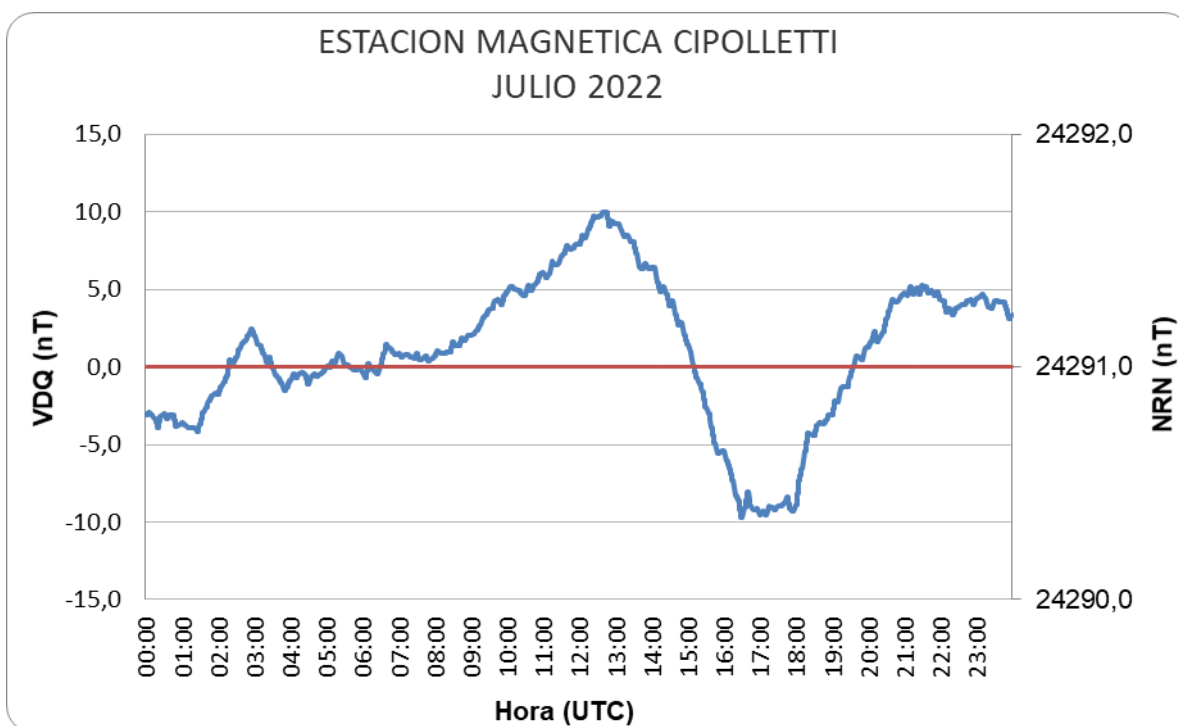
Figura 7: Variación Diaria Calma del mes de julio
