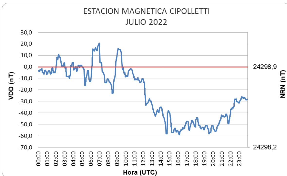
Figura 8: Variación Diaria Perturbada del mes de julio
