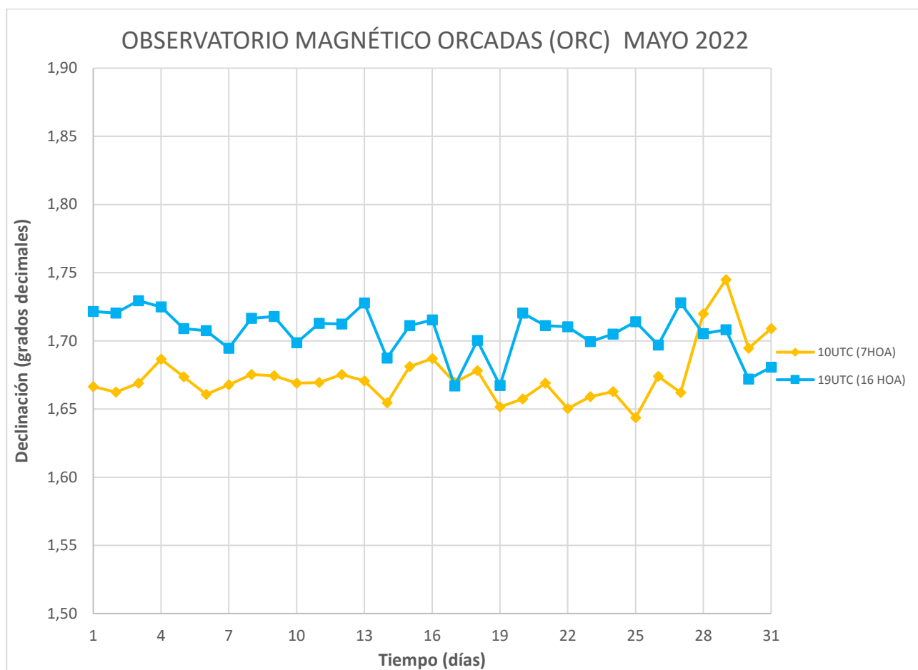
Figura 5: Declinación magnética en función del tiempo
