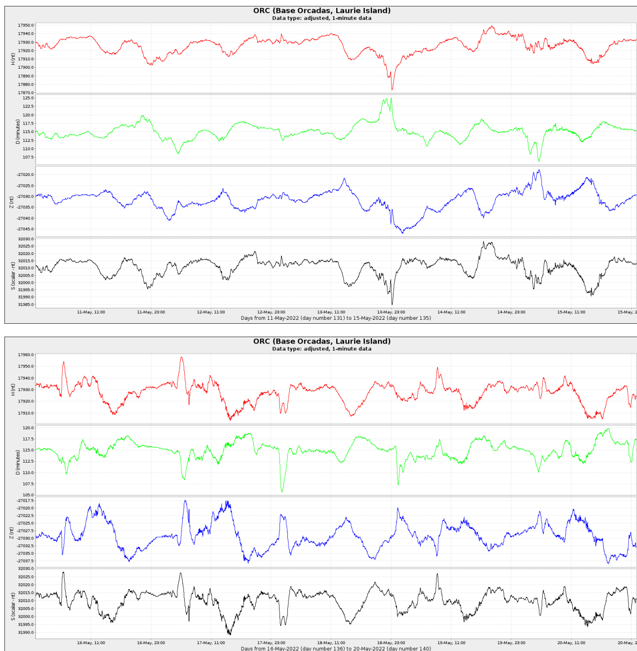
Figura 4b Componentes del campo magnético del 11 al 20 de mayo. En rojo se ve la componente horizontal (H) y en azul la vertical (Z), ambas en nT. En verde se presenta la declinación del campo magnético (D) en minutos y en negro la intensidad del campo magnético en nT.
