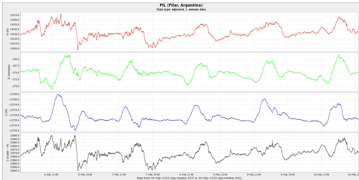
Figura 4a: Componentes del campo magnético del día 1al 10 de febrero. En rojo se ve la componente horizontal (H) y en azul la vertical (Z), ambas en nT. En verde se presenta la declinación del campo magnético (D) en minutos y en negro la intensidad del campo magnético en nT
